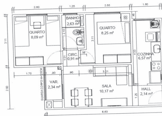
TIPOLOGIA TIPO (2º AO 11º PAVIMENTOS)
