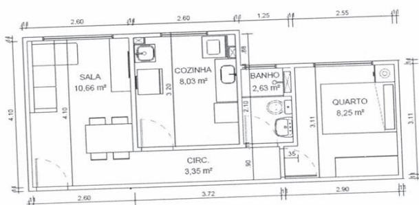
TIPOLOGIA TÉRREO (SEM ÁREA PRIVATIVA) TORRES 01 E 02 METRAGEM DAS ÁREAS PRIVATIVAS DO APARTAMENTO = 37,28m² 04 UNIDADES HABITACIONAIS NO TOTAL
