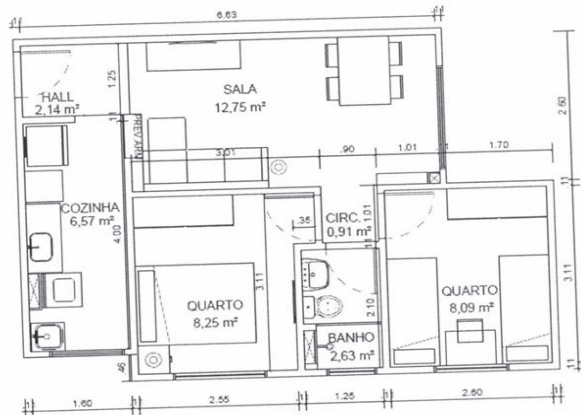
TIPOLOGIA TÉRREO (SEM ÁREA PRIVATIVA) TORRES 01 E 02 METRAGEM DAS ÁREAS PRIVATIVAS DO APARTAMENTO = 45,64m² 01 UNIDADE HABITACIONAL NO TOTAL
