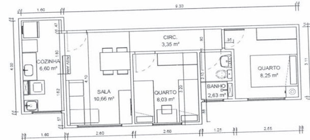
TIPOLOGIA TIPO (2º AO 11º PAVIMENTOS) TORRES 01 E 02 METRAGEM DAS ÁREAS PRIVATIVAS DO APARTAMENTO = 44,32m² 76 UNIDADES HABITACIONAIS NO TOTAL
