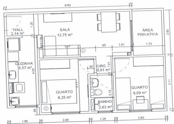
TIPOLOGIA TÉRREO (COM ÁREA PRIVATIVA)
