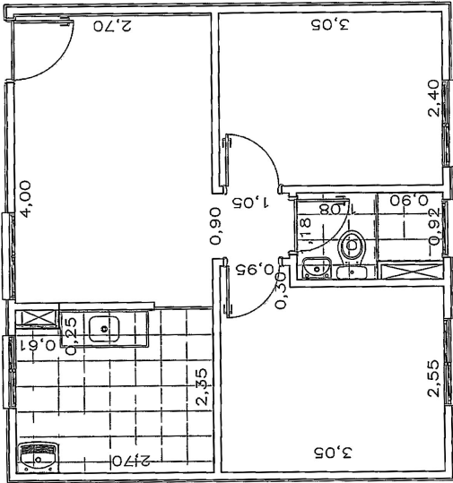
LAYOUT - APTO. TIPO 3 ESCALA 1:50
