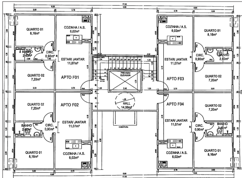
PLANTA PAV. TIPO - BLOCOS 01 A 17
