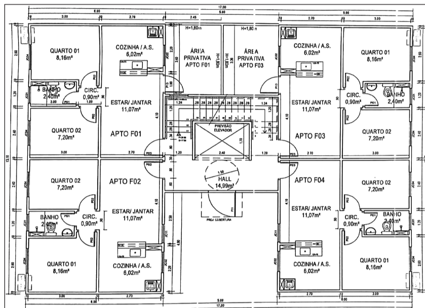
PLANTA PAV. TÉRREO - BLOCOS 01 A 17
