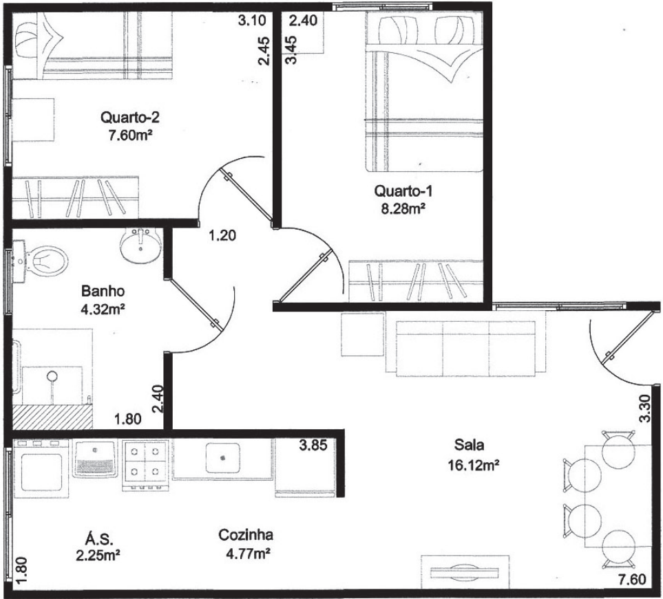
PLANTA APARTAMENTO TÉRREO E TIPO ÁREA CONSTRUÍDA 47,50 M²
