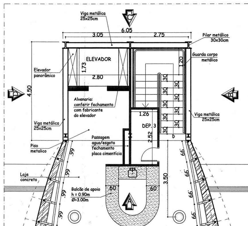
PLANTA BAIXA SUPERIOR
