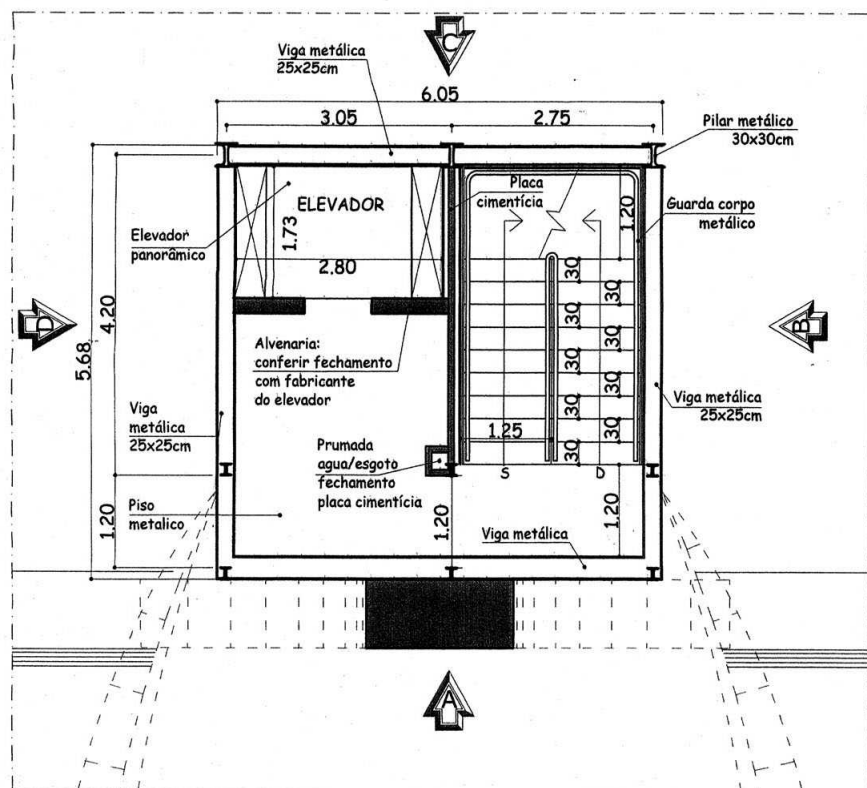
PLANTA BAIXA PAV. TIPO COM ACESSO ELEVADOR
