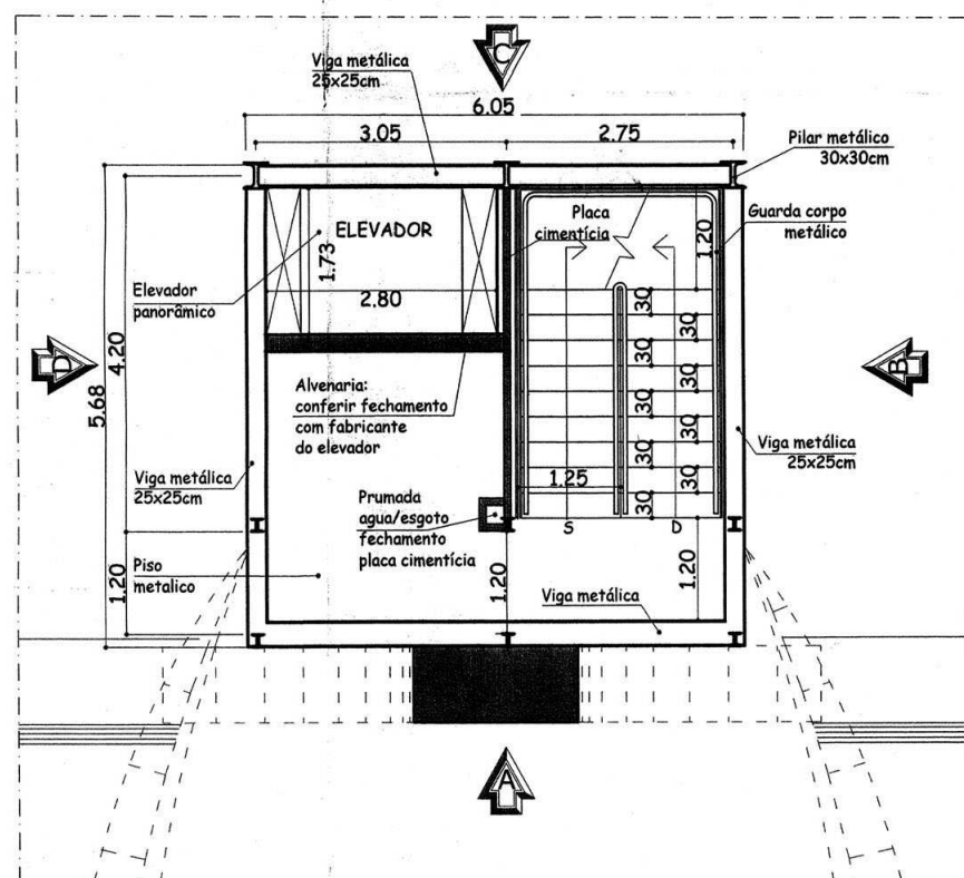
PLANTA BAIXA PAV. TIPO SEM ACESSO ELEVADOR
