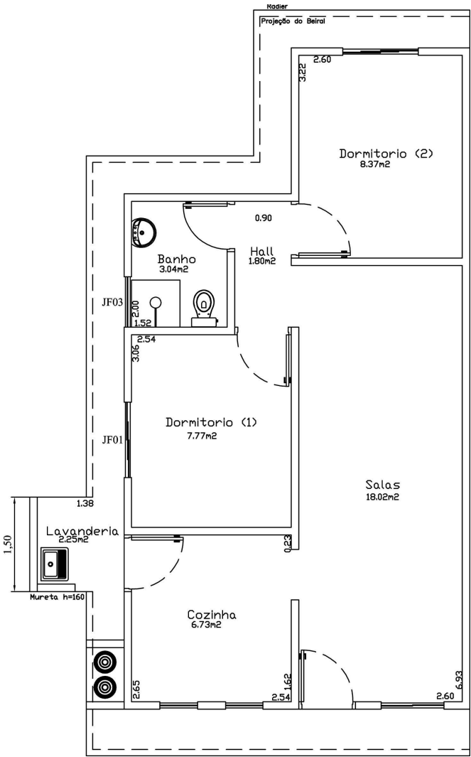
PLANTA BAIXA (MODELO CTG-2Q-7-57D)
