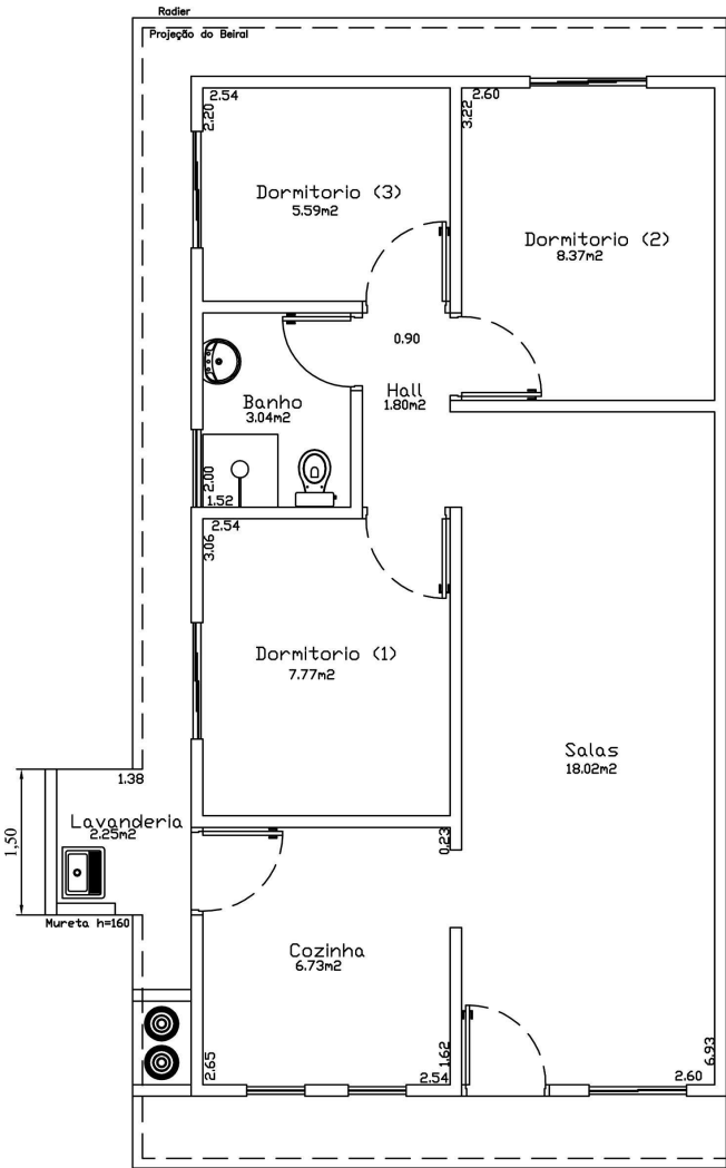
PLANTA BAIXA (MODELO CTG-3Q-7-60D)
