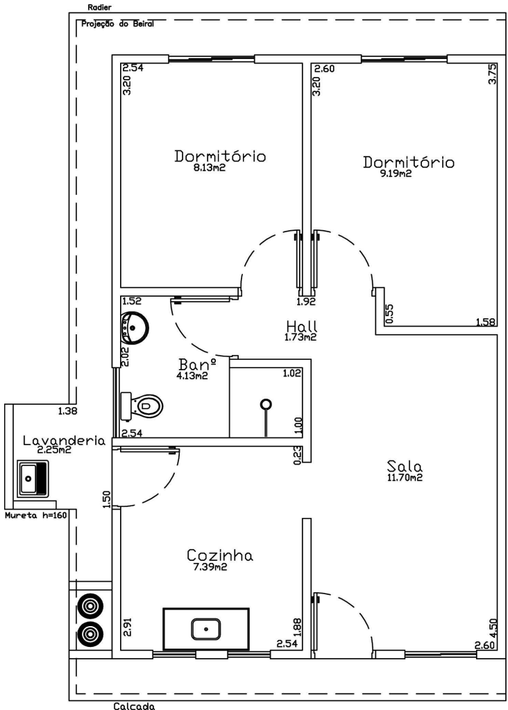
PLANTA BAIXA (MODELO CTG-2Q-7-50D)
