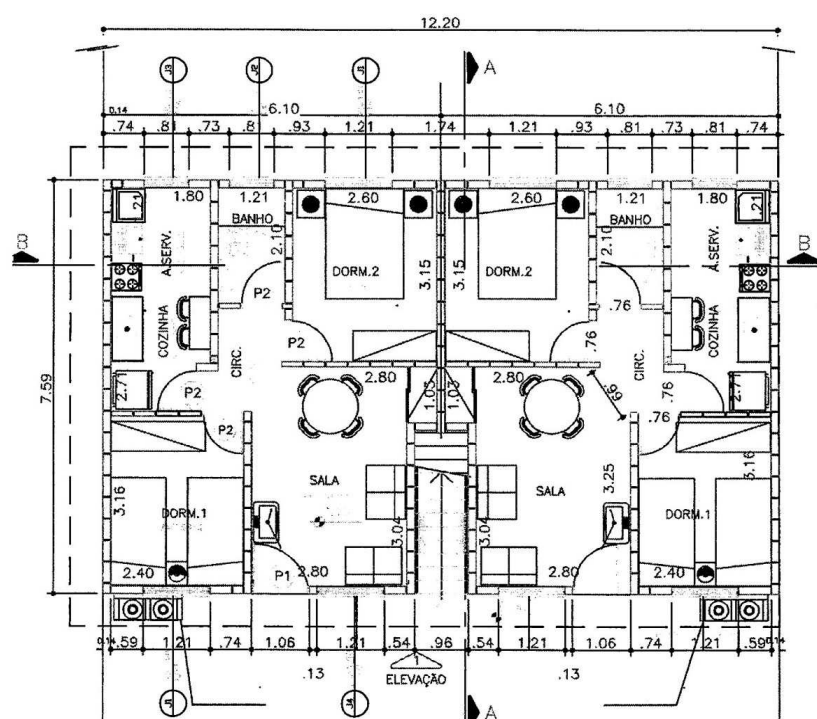
PLANTA - PAV. TÉRREO ESCALA 1:100
