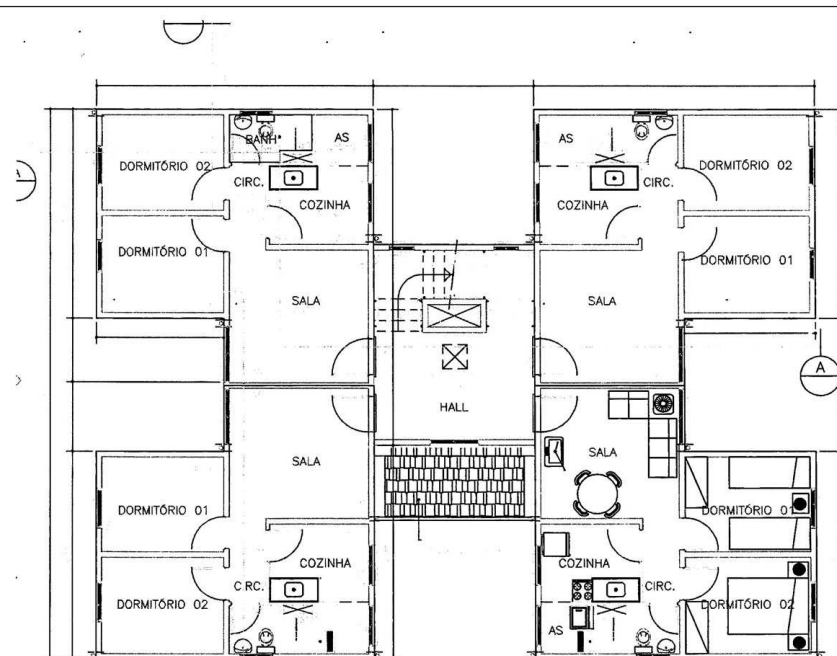
PLANTA PAVIMENTO TIPO ESC.: 1:100
