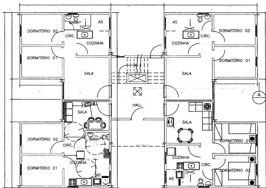
PLANTA PAVIMENTO TÉRREO - APTO. ADAPTADO ESC.: 1:100 APTO. 11 - BLOCOS 01,04,05,08,11,12,13,15,19,22,23,25,26
