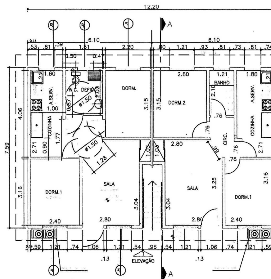
PLANTA - PAV. TÉRREO - ADAPTADO ESCALA 1:100 APTO. 11 - BLOCOS: 01, 04, 05, 20, 31, 42, 51
