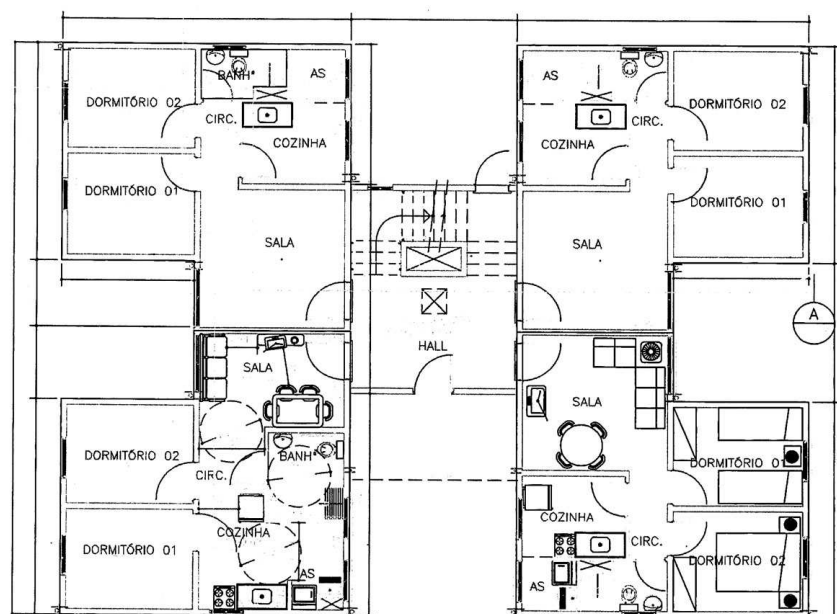
PLANTA PAVIMENTO TÉRREO - APTO. ADAPTADO ESC.: 1:100 APTO. 11 - BLOCOS: 01, 05, 07, 08, 12, 13, 14, 15, 19, 20, 24, 25, 29, 30
